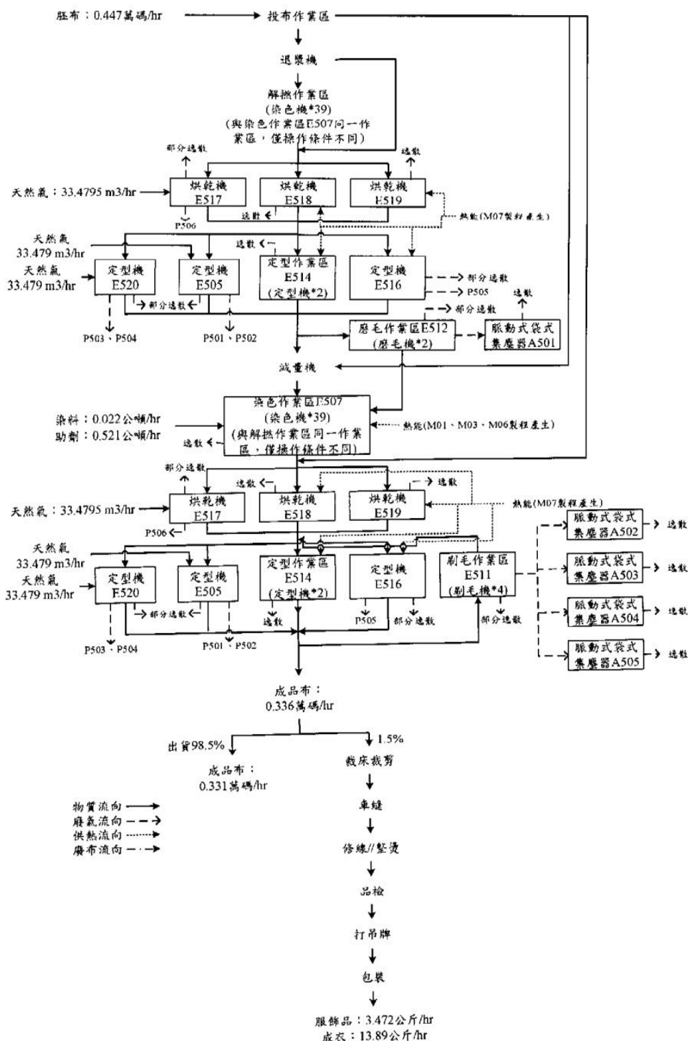
圖6、M05製程流程圖例
