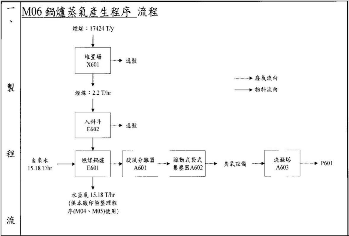
圖7、M06製程流程圖例
