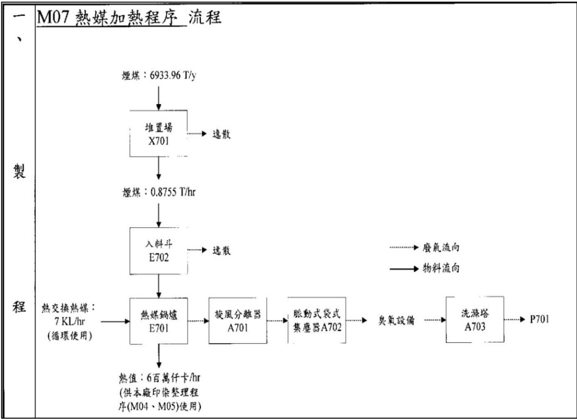
圖8、M07製程流程圖例
